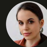
Ольга Михайлюк
